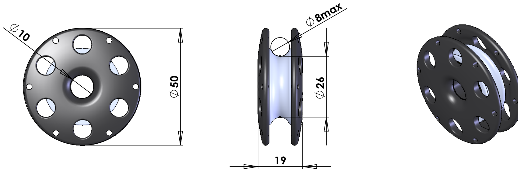
Self-lubricating plain bearings block Poulie à roulement à palier auto-lubrifié
