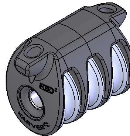
Balls-bearing block Poulie à billes
