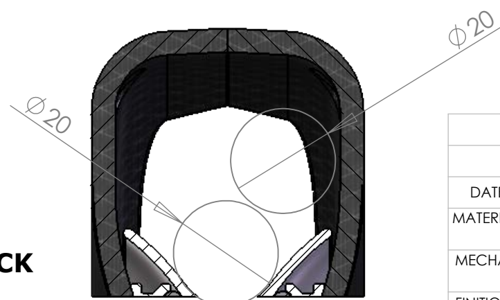
COUPE D-D ECHELLE 1 : 1
